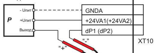
Датчик давления
