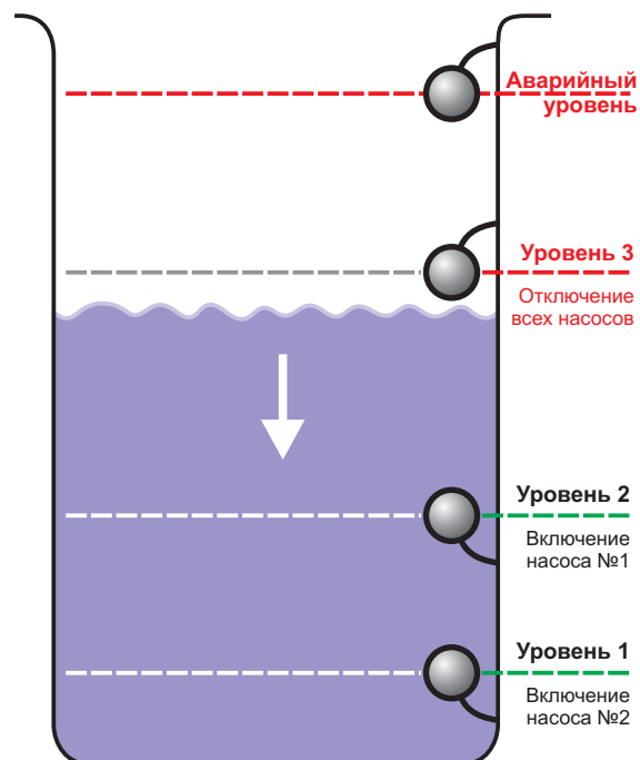
2 рабочих насоса
