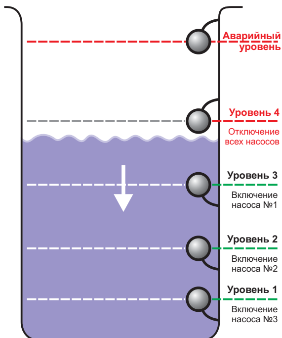
3 рабочих насоса
